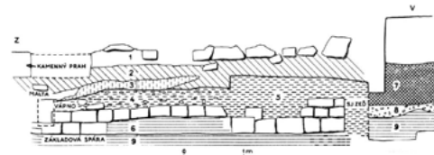
Severní stěna kvádríkového objektu. Původní kresebná dokumentace Václava Humla. © Muzeum hlavního města Prahy
