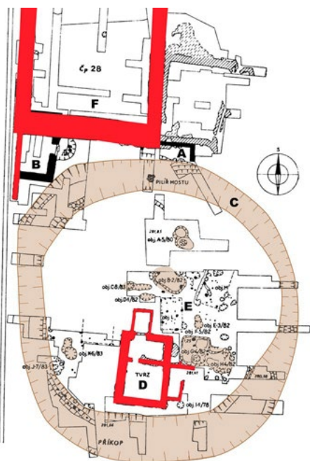
Celkový plán tvrziště a souvisejících nálezů. A – torzo starší kamenné kvádríkové stavby; B – torzo starší stavby z lomového zdiva; C – kruhový příkop mladší tvrže porušující starší stavby; D – kamenný suterén věžové tvrže; E – pozůstatky dřevohlinitých staveb; F – hospodářský dvůr. Podle Václava Humla. © Muzeum hlavního města Prahy
