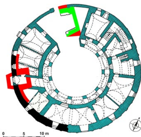
Půdorys přízemí tvrze podle zaměření Státního ústavu pro rekonstrukci památkových měst a objektů. Černě, červeně a zeleně jednotlivé gotické fáze. Modře mladší nerozlišené fáze. Podle V. Humla. © Muzeum hlavního města Prahy
